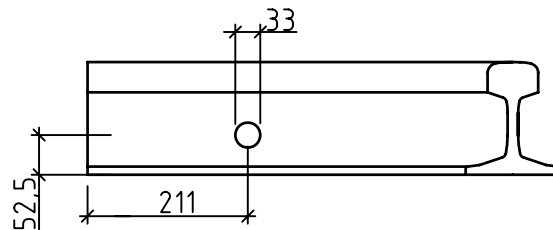
Detalj hålning för skarvjärn Skala 1:10
